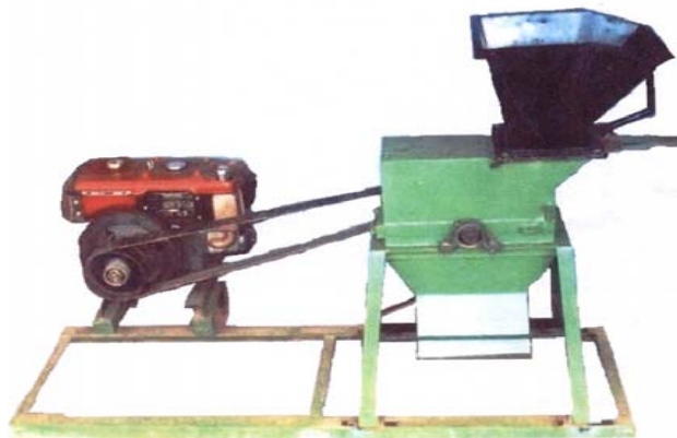
Broyeur Polyvalent Motorisé pour produits d'agriculture et d'élevage/Oumar Tibila ROUAMBA
